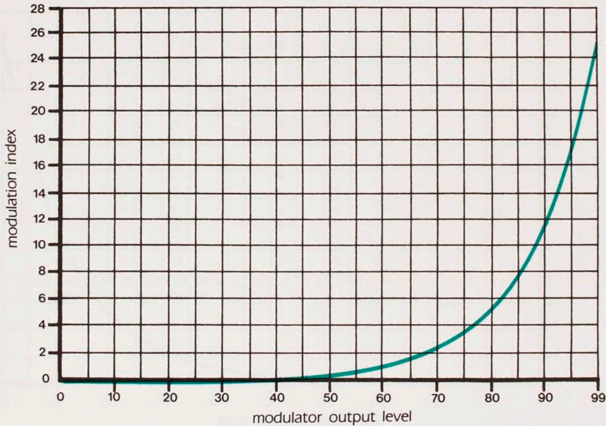
DX21——Index vs. Output Level
